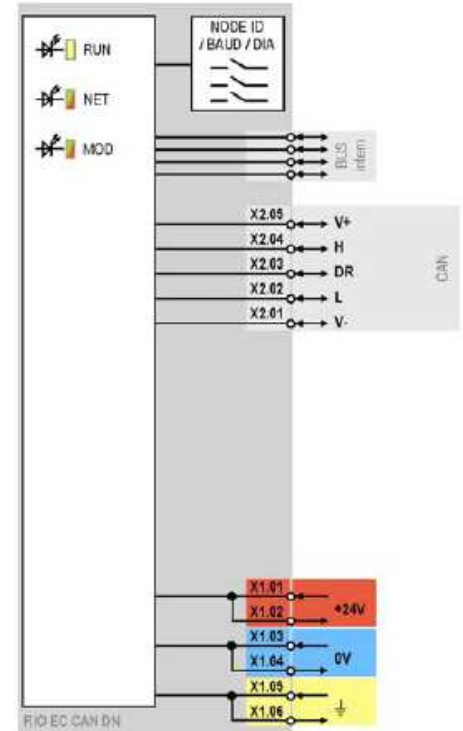
schemat blokowy
